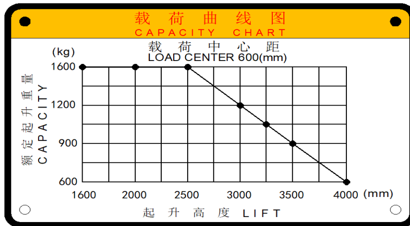
Load chart CDD16-EMT-J
