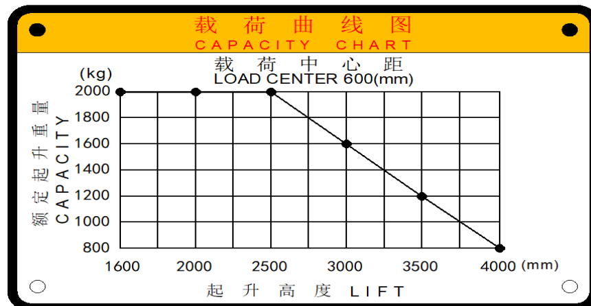
Load chart CDD20-EMT-J
